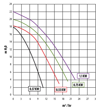
CURVAS DE RENDIMENTO / BOMBA STA-RITE 5P2R
