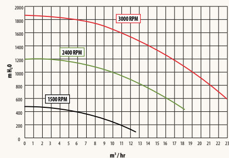
CURVAS DE RENDIMENTO / BOMBA RS II® VSTD
