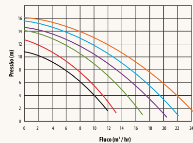
CURVAS DE RENDIMENTO / BOMBA POWERLINE PL
