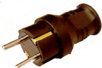
Clavija de goma Macho Ø4,8mm 16A/250V~ mevi.1183
