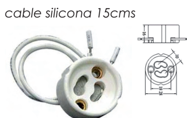
Portalámparas GU10/GZ10 mevi. 4080
