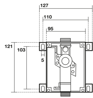
7565 Dispositivo di cacciata a parete per orinatoio Concealed urinal flush valve
