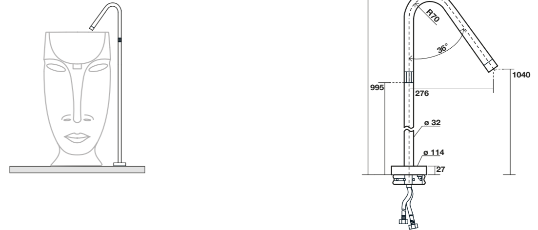
7562 Bocca di erogazione per orinatoio Groove inox satinato Stainless steel satin floor mounted spout for orinal Groove
