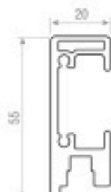
Guía superior
