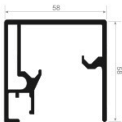
Guía superior
