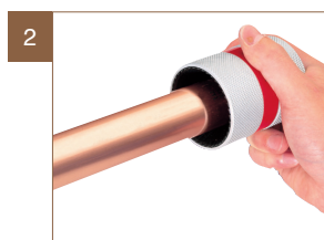
Desbarbar y calibrar el tubo
