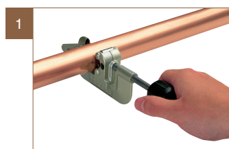
Cortar el tubo
