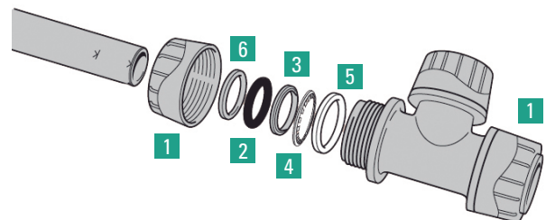
Configuración general de los accesorios
