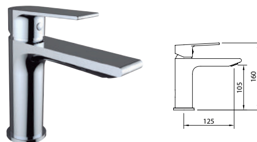
LAVABO 105 Basin mixer 105 | Mitigeur lavabo 105 Mezclador con aireador y flexibles M-10 3/8" x 420 mm. Mixer, aerator, flexible hoses M-10 3/8" x 420 mm. Mitigeur Lavabo, aérateur, raccords flexibles M-10 3/8" x 420 mm
