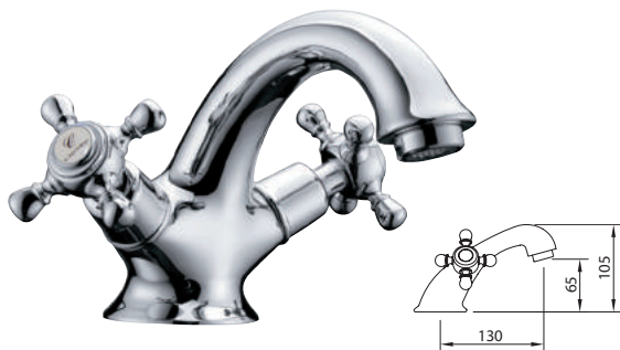
LAVABO 65 Basin mixer 65 | Mélangeur lavabo 65
