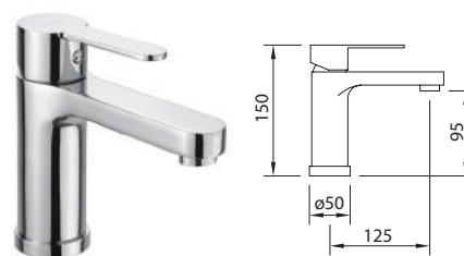
LAVABO 95 Basin mixer 95 | Mitigeur lavabo 95
