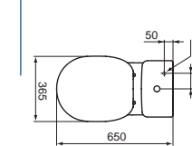
Esquema con salida dual para instalación con tanque cúbico
