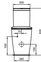
Esquema con salida dual para instalación con tanque angular
