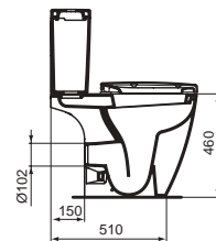
Esquema con salida dual para instalación con tanque cúbico
