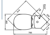
Esquema con salida dual para instalación con tanque angular
