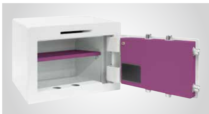
Bulones guiados por soportes macizos y alojamiento interno para bulones.
