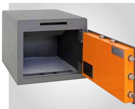
Bulones giratorios y guiados que impiden su corte desde el exterior. Alojamiento interno para bulones.
