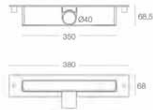
Válvula lineal. Evacuación 0,6 lts/seg., atornillada, vaso sifón
