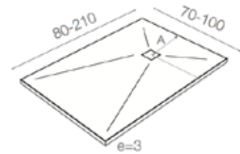
Cotas desagüe
