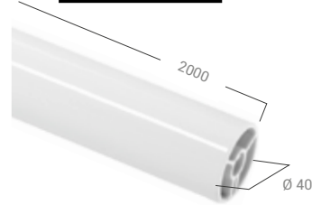
Alumínio termolacado branco, RAL9016. Aluminio, fundición de aluminio termo- lacado blanco RAL 9016
